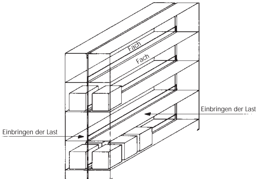
Abb. 9 a: 4 Fächer = Feld eines Einfachregals
