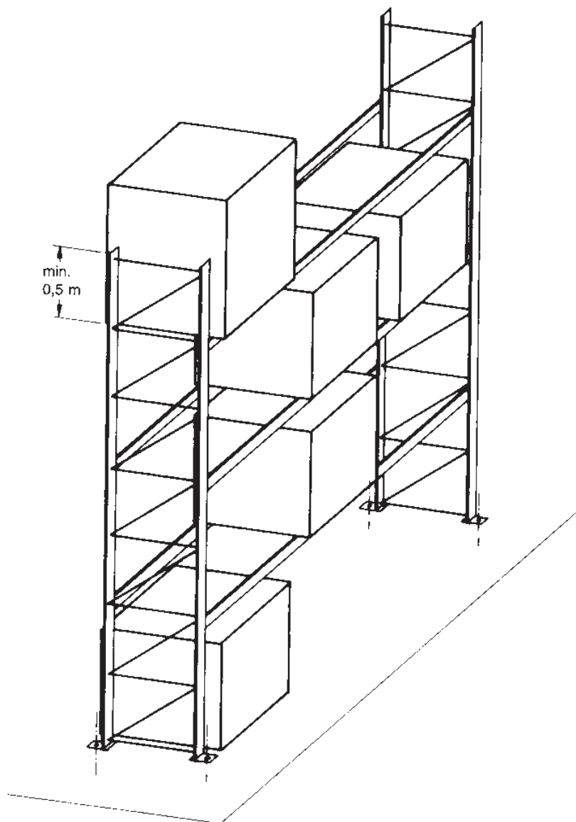
Abb. 7: Beispiel einer Sicherung gegen seitliches Herabfallen der Ladeinheiten.
