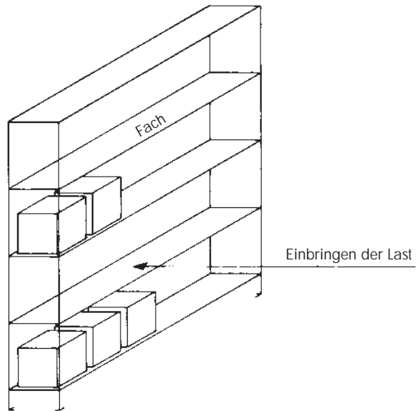
Abb. 9 a: 4 Fächer = Feld eines Einfachregals
